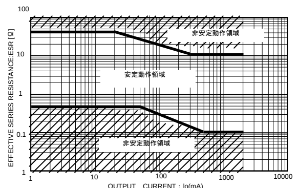
Fig.34 ESR vs I_o 特性 (BAxxDD0, 22μF)
