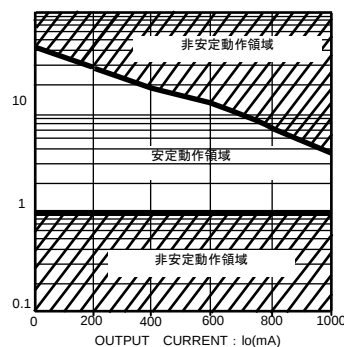
Fig.33 ESR - I_o 特性 (BAxxCC0, 22μF)
