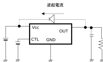
Fig.35: バイパスダイオード
