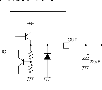
Fig.32 出力等価回路
