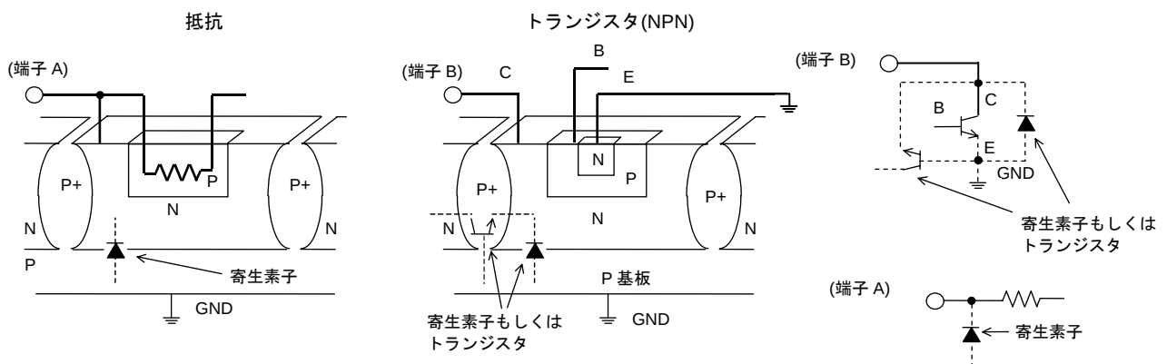
Fig.36 バイポーラ IC の構造例
